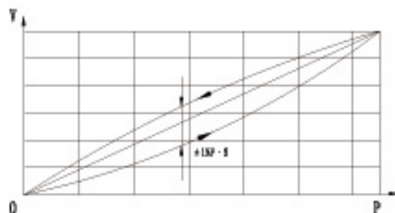
典型静态校准误差曲线
